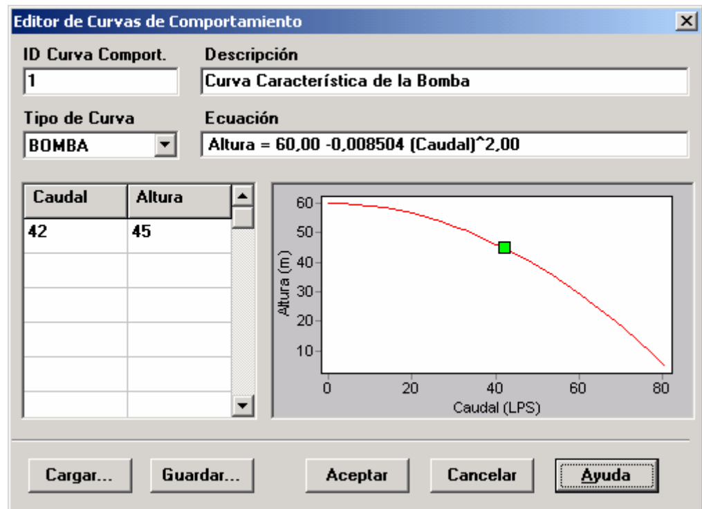
Figura 6.1 Editor de Curvas de Comportamiento
