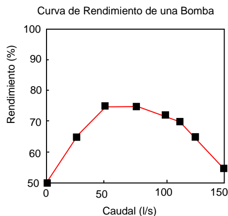
Figura 3.3 Curva de Rendimiento de una Bomba
