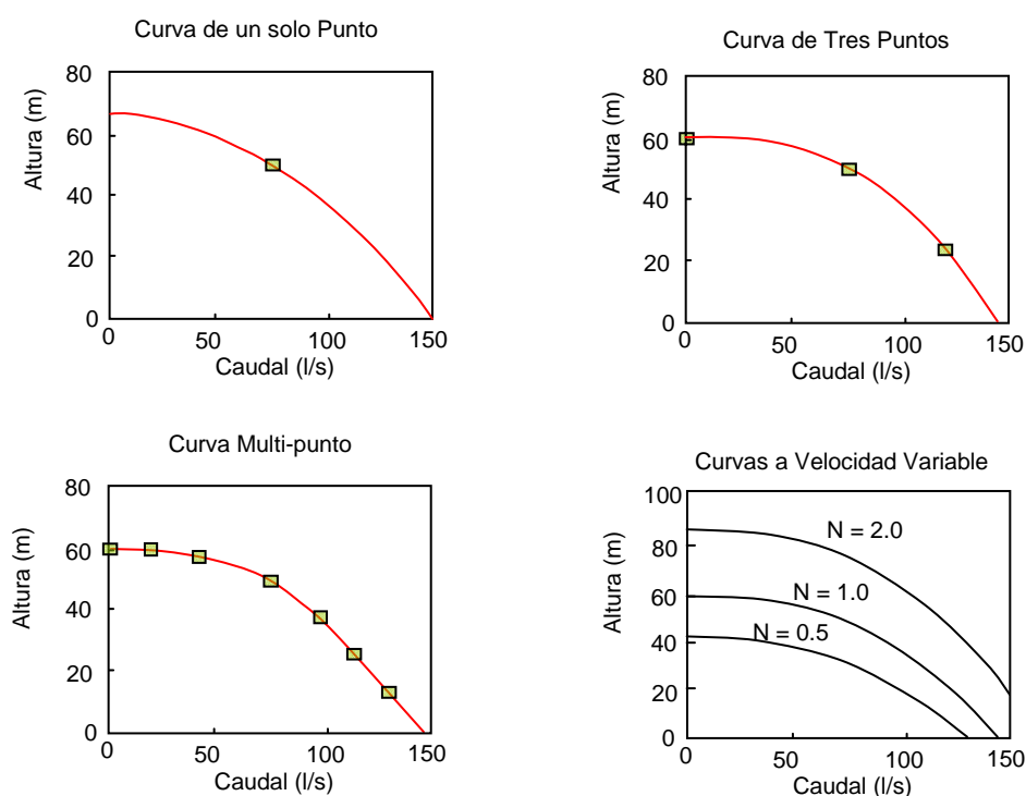
Figura 3.2 Ejemplos de Curvas Características de una Bomba
